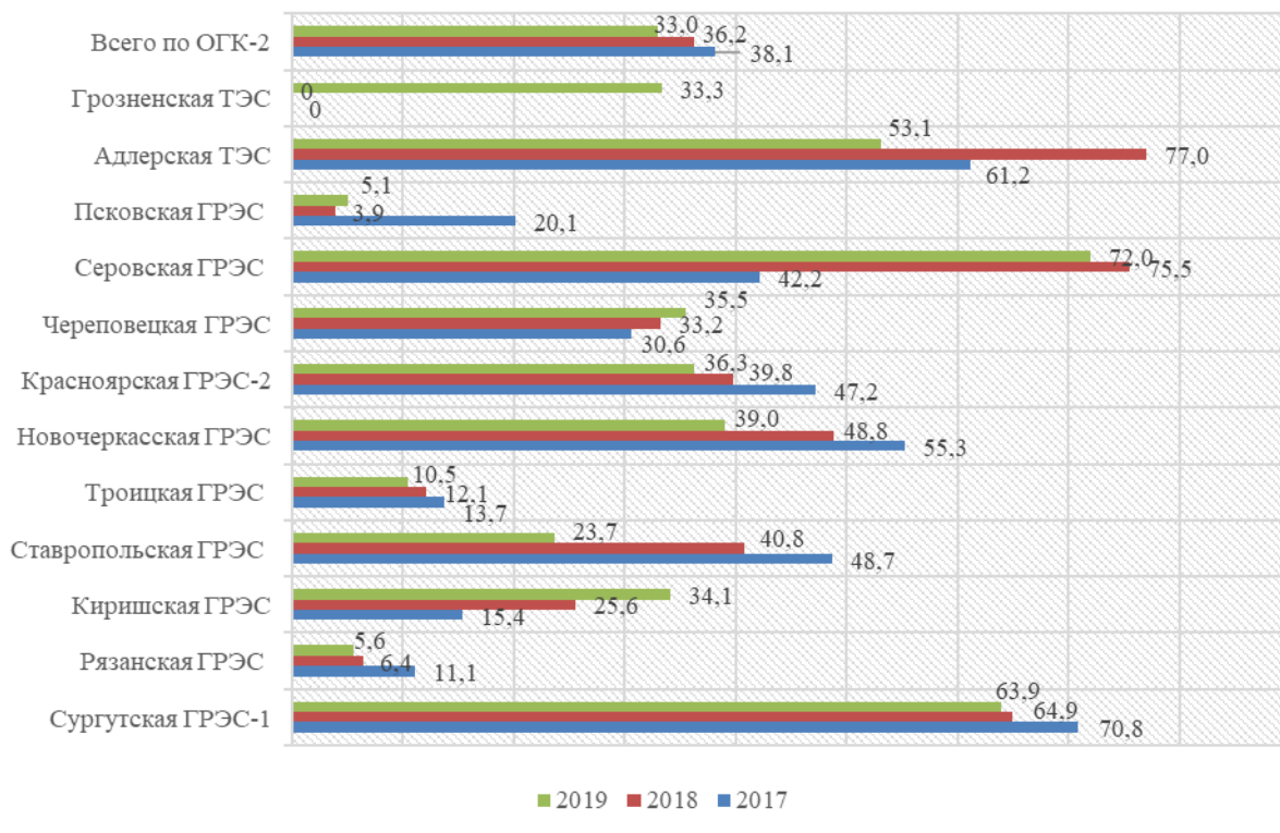
Динамика изменения КИУМ станций ОГК-2 в 2017-2019 гг., %
