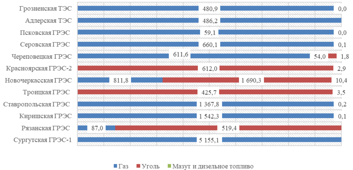
Структура и фактический расход топлива на электростанциях ОГК-2 в 2020 году, тыс. тунт
