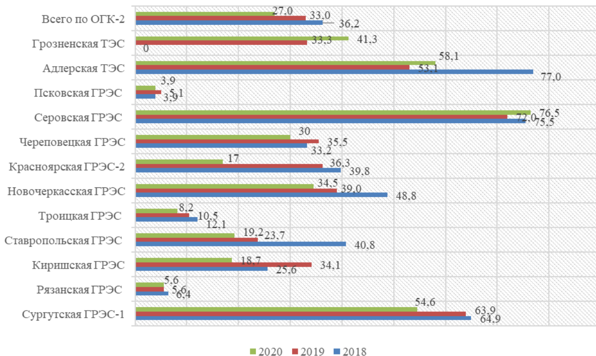
Динамика изменения КИУМ станций ОГК-2 в 2018-2020 гг., %
